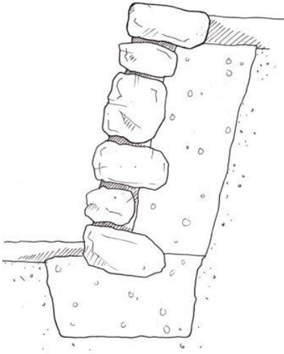
Trockenmauer im Querschnitt
